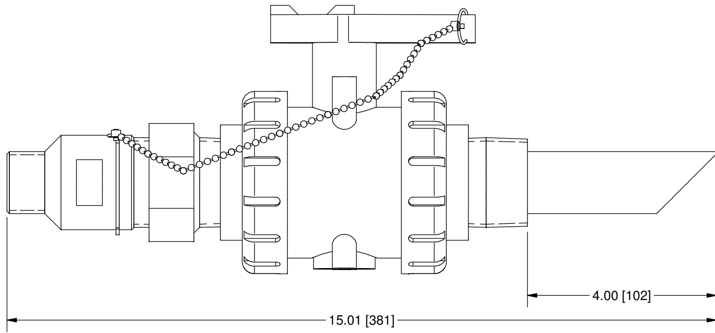
SCALE 1 : 2
