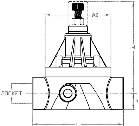
Socket
