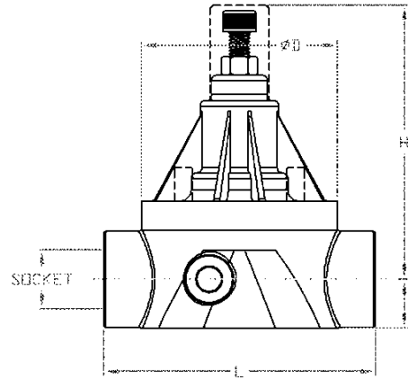
Socket
